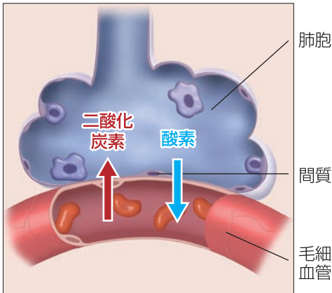
正常肺構造
